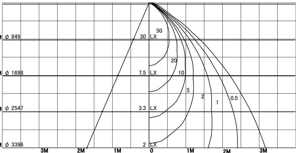
1/2照度角
