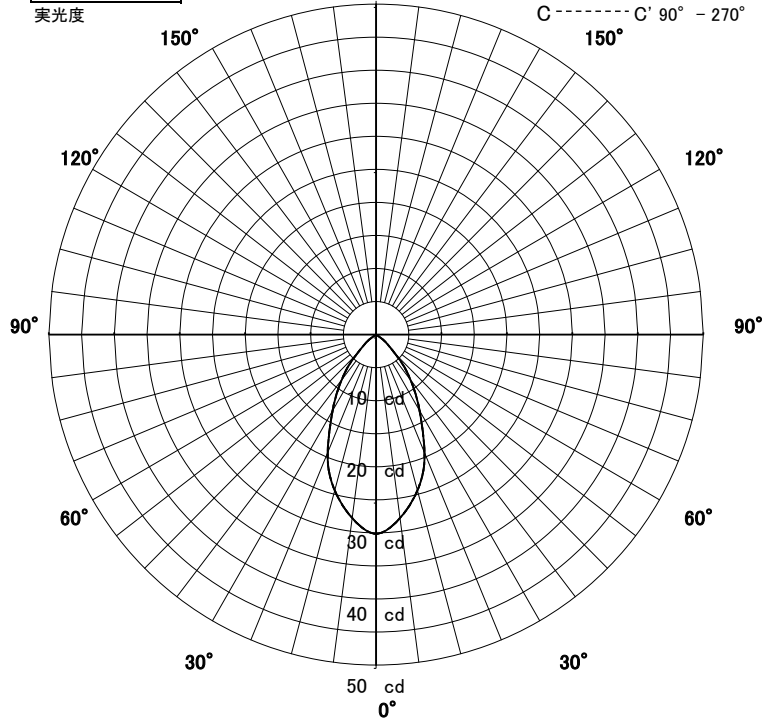
配光曲線図
